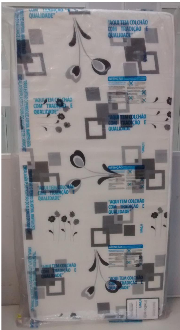
FOTO 1: AMOSTRA RECEBIDA PARA ENSAIO
